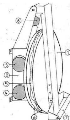
Bild 6. Bälgs 1. Bälglock 2. Ventilhus 3. Blindlock (insug) 4. Blindlock (utblåsning) 5. Bälgtyg 6. Slangklämma 7. Handtag 8. Reparationsatts
